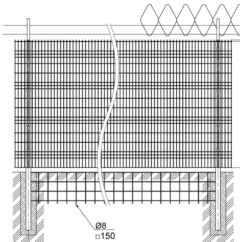
Рисунок 14 – Крепление противоподкопного барьера
